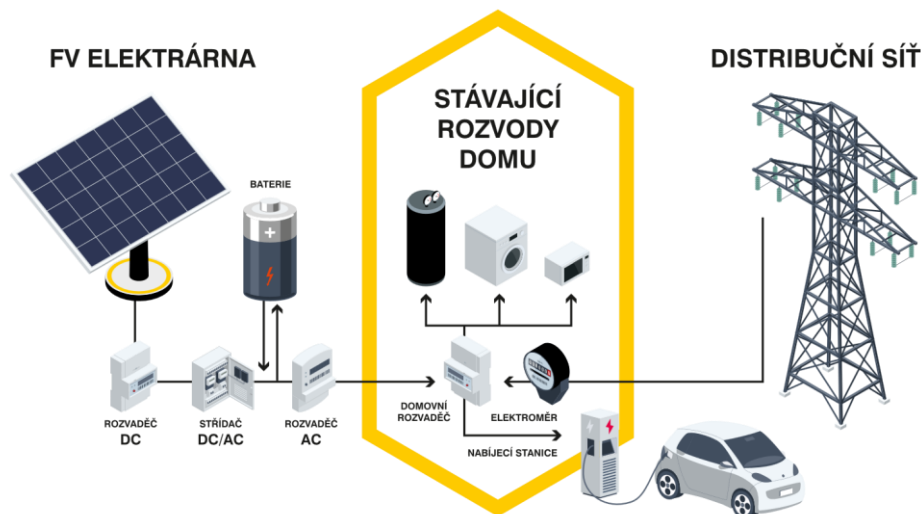
Ukázka hybridní fotovoltaická elektrárny
